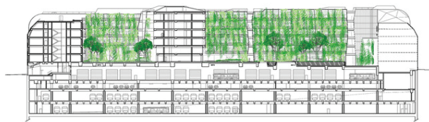
Paris Pyrénées - Coupe longitudinale © Métra et associés
